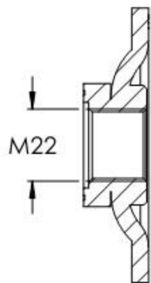
SCHNITT A-A
