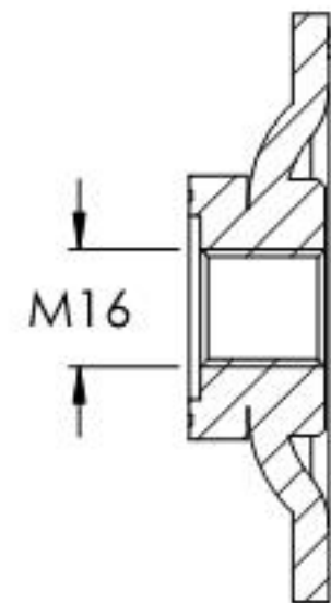
SCHNITT A-A
