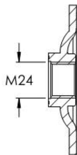
SCHNITT A-A
