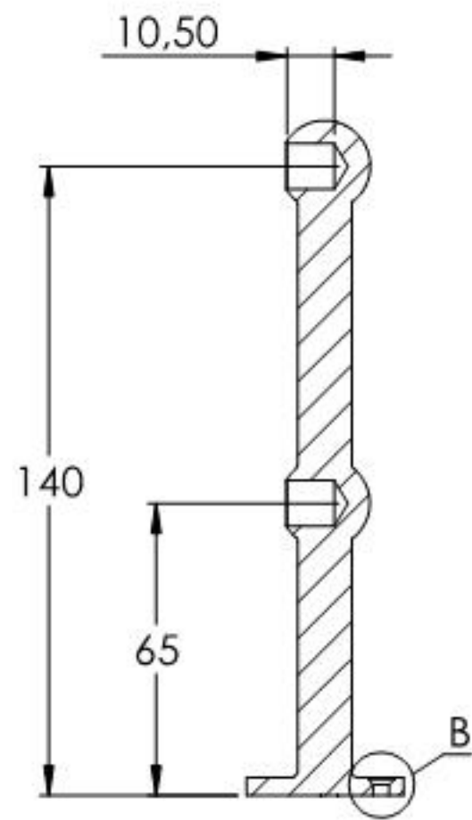
SCHNITT A-A
