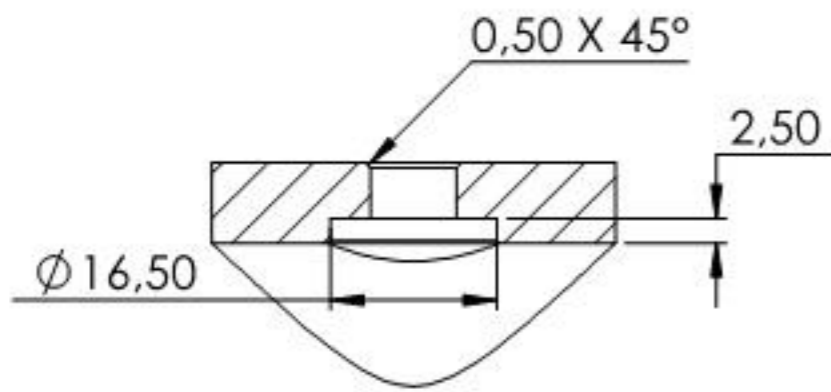
SCHNITT C-C
