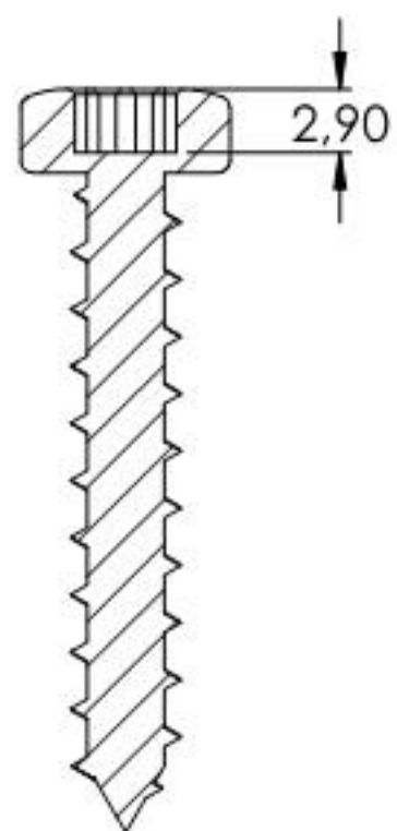
SCHNITT A-A
