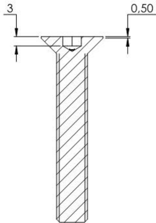
SCHNITT A-A
