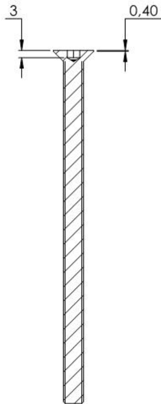
SCHNITT A-A
