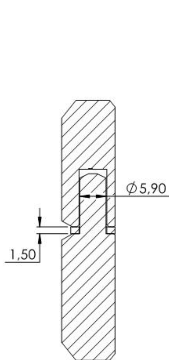
SCHNITT A-A
