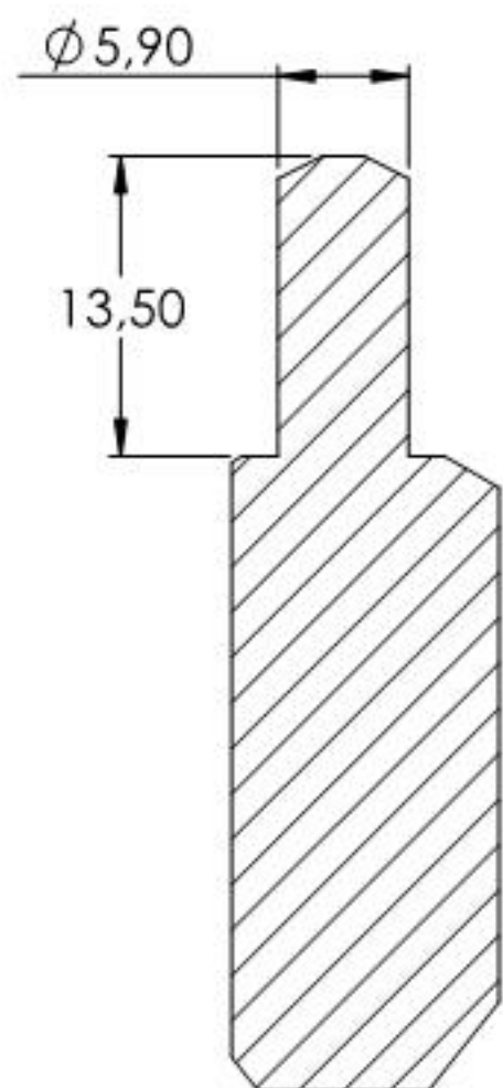
SCHNITT C-C
