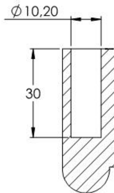
SCHNITT B-B
