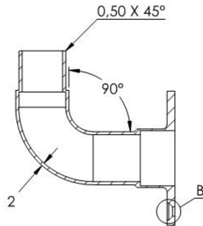
SCHNITT A-A
