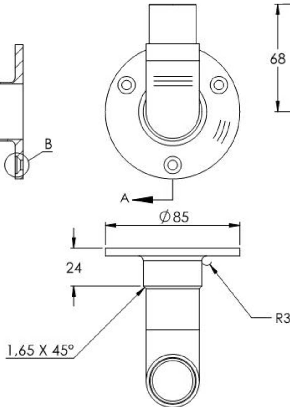
SCHNITT A-A
