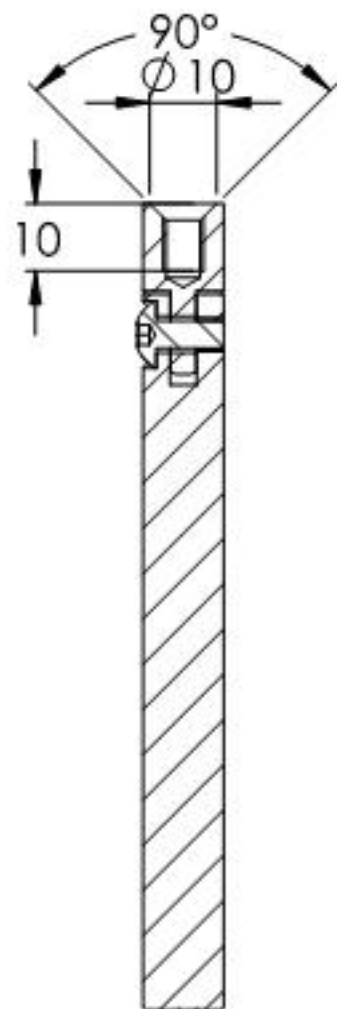
SCHNITT A-A
