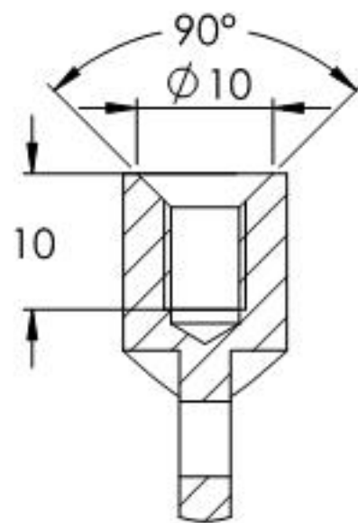
SCHNITT C-C
