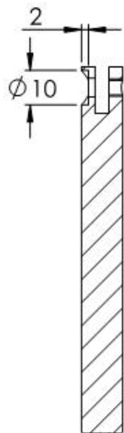
SCHNITT B-B
