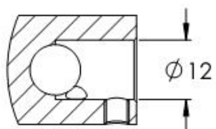
SCHNITT A-A
