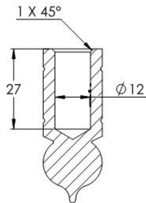
SCHNITT C-C
