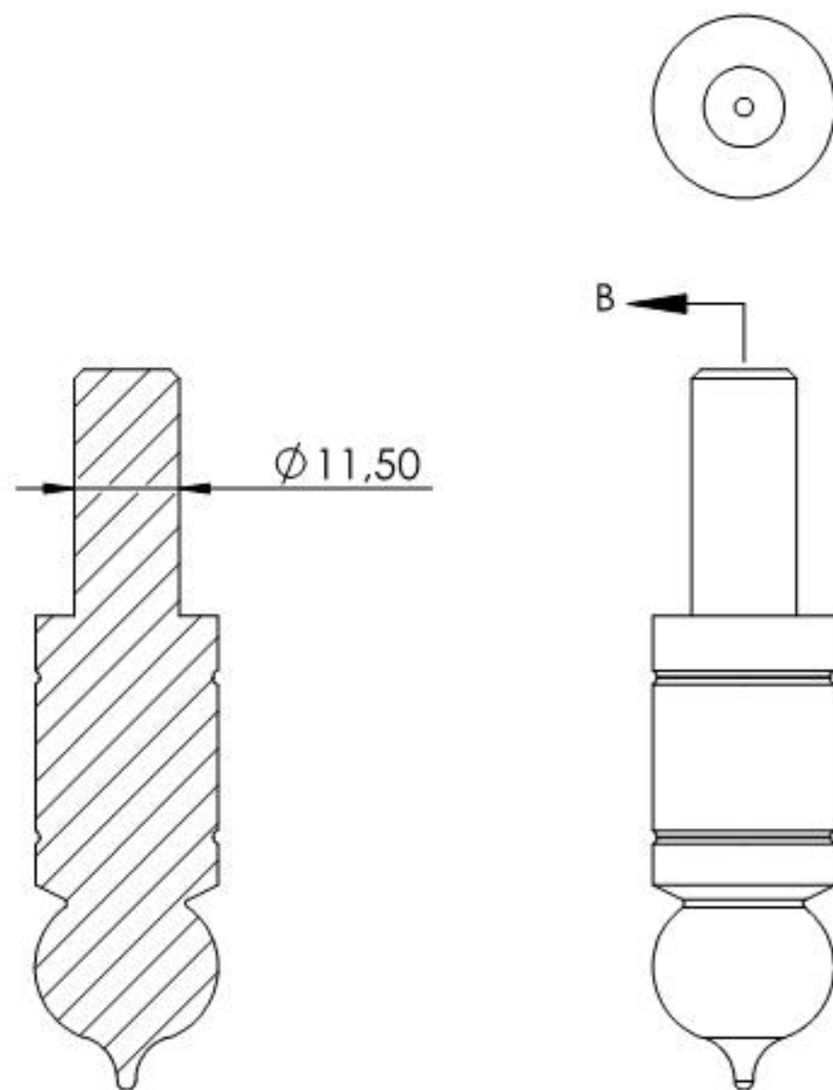
SCHNITT B-B
