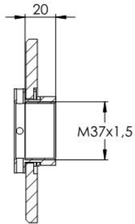
SCHNITT A-A
