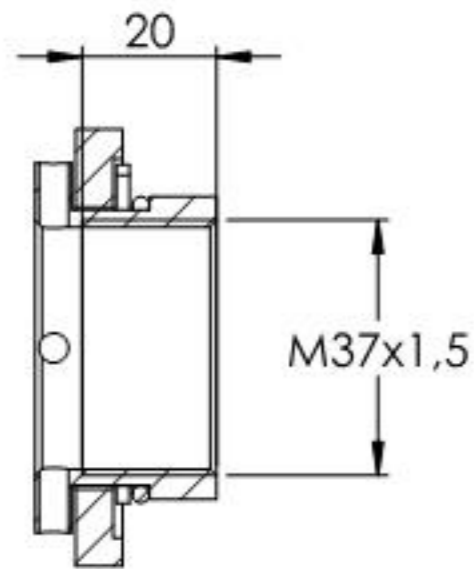
SCHNITT A-A
