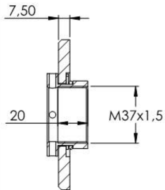
SCHNITT A-A
