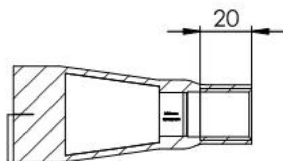
SCHNITT A-A
