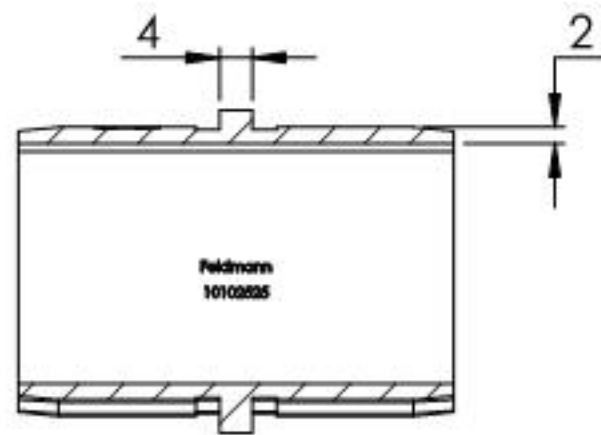
SCHNITT A-A
