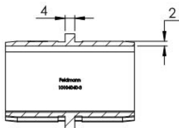
SCHNITT A-A
