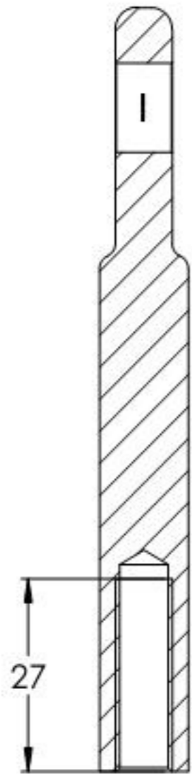
SCHNITT A-A
