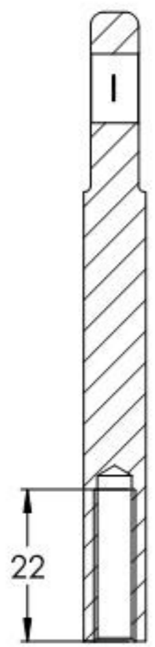
SCHNITT A-A
