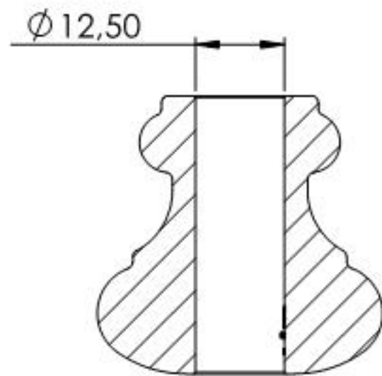
SCHNITT A-A
