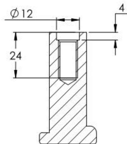
SCHNITT B-B
