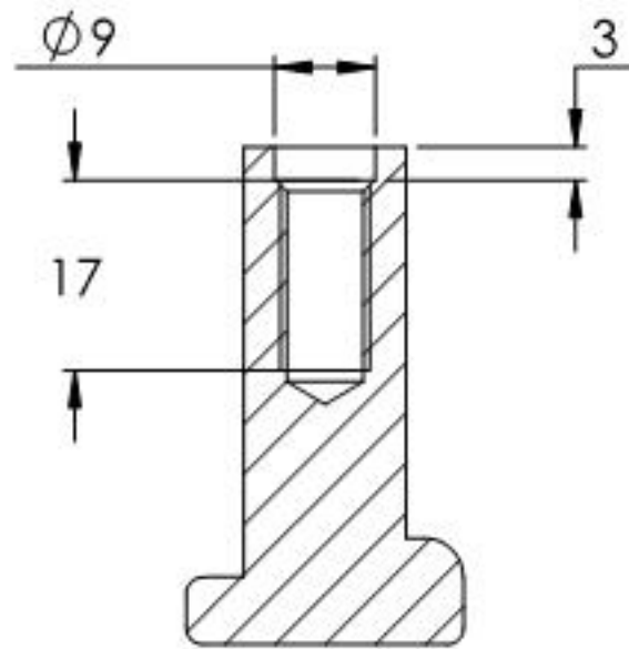
SCHNITT B-B
