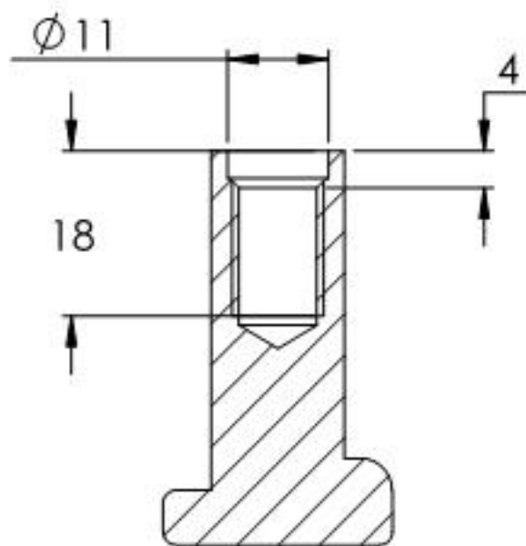
SCHNITT B-B
