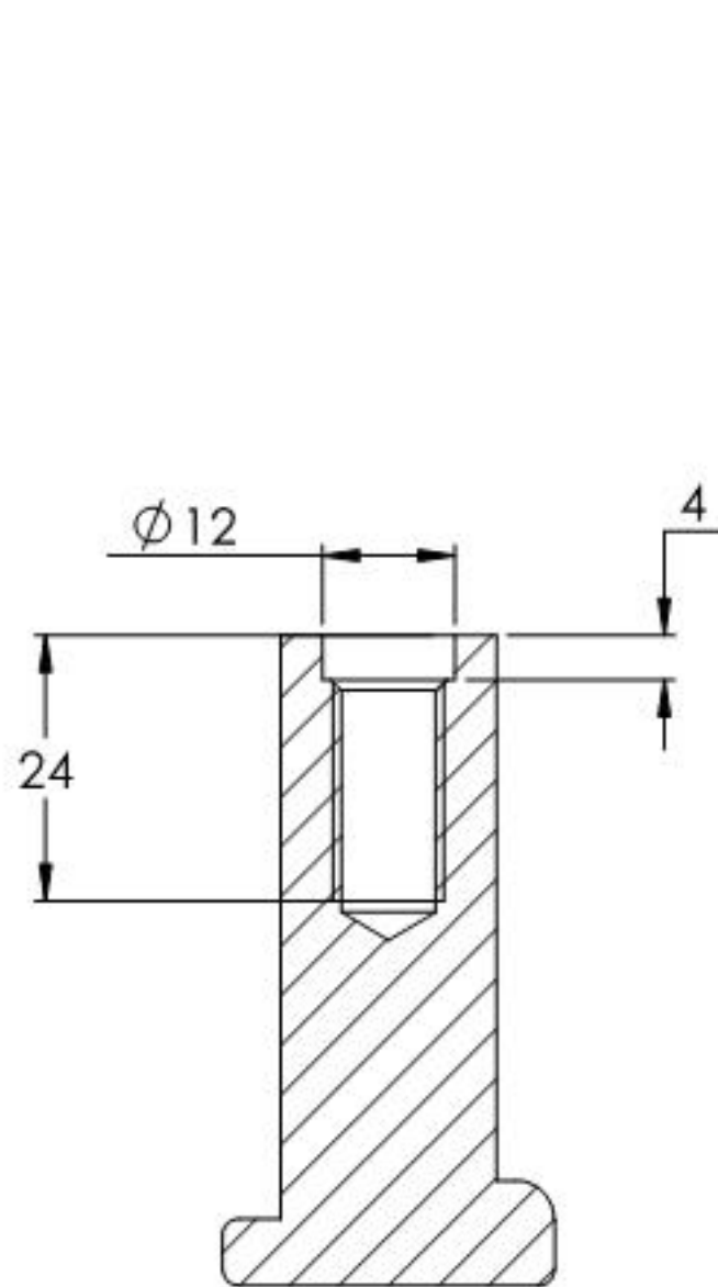
SCHNITT B-B
