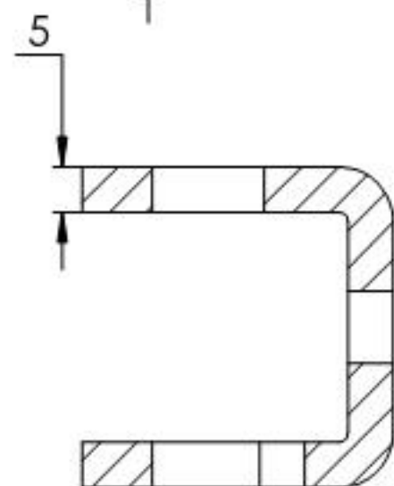
SCHNITT A-A
