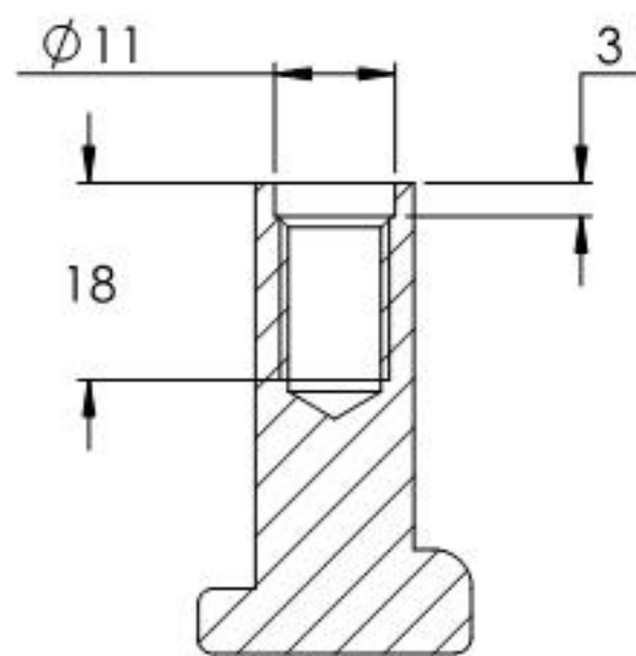
SCHNITT B-B
