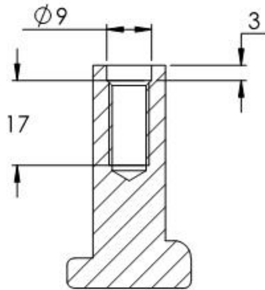
SCHNITT B-B
