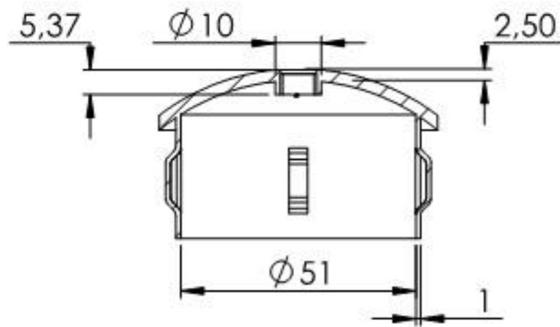
SCHNITT A-A
