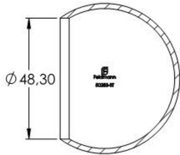
SCHNITT A-A
