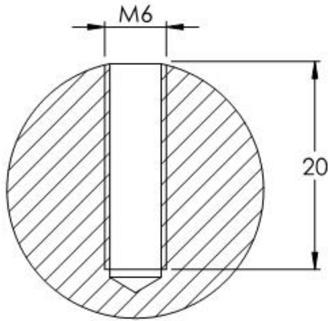
SCHNITT A-A
