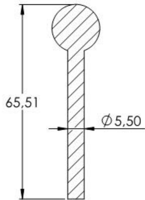
SCHNITT A-A
