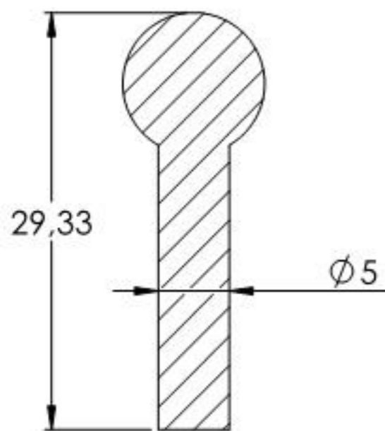
SCHNITT A-A
