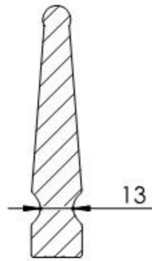
SCHNITT A-A
