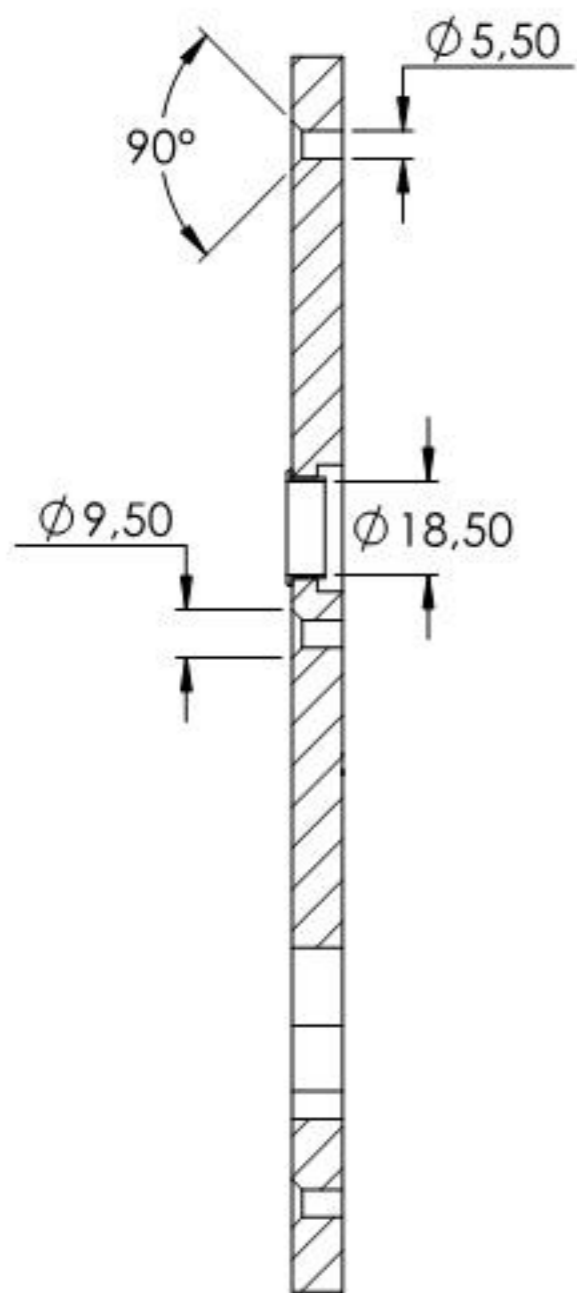
SCHNITT A-A
