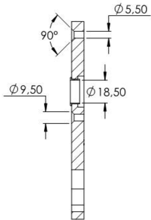
SCHNITT A-A
