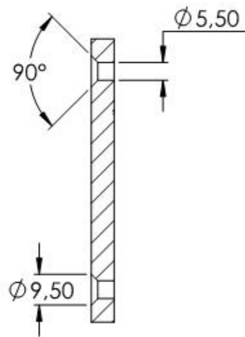
SCHNITT A-A
