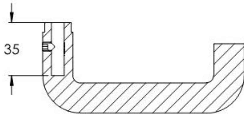
SCHNITT A-A
