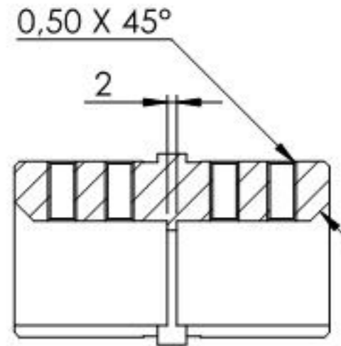
SCHNITT A-A
