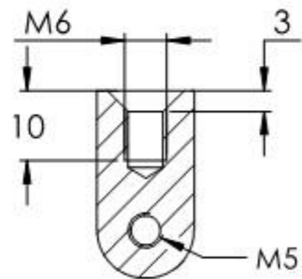
SCHNITT C-C
