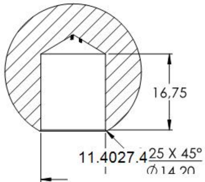
SCHNITT A-A
