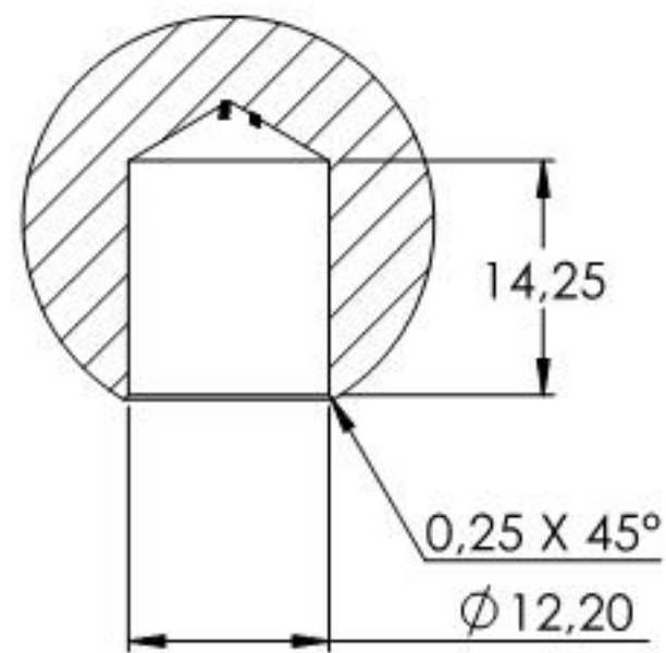
SCHNITT A-A
