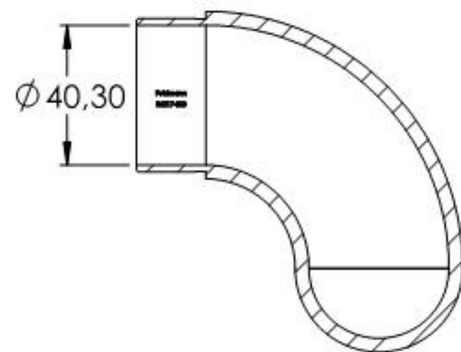
SCHNITT A-A
