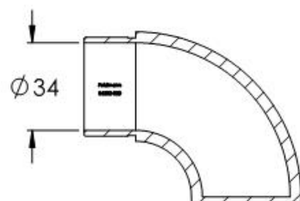
SCHNITT A-A
