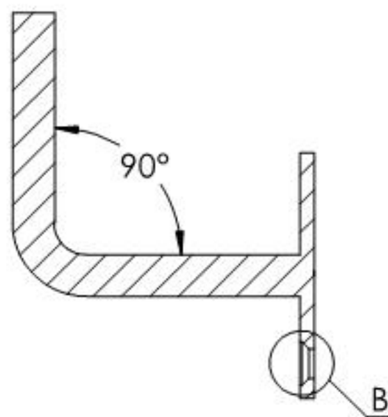
SCHNITT A-A
