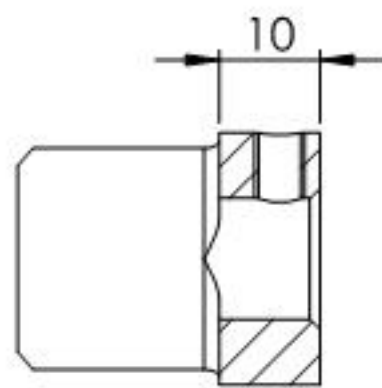
SCHNITT B-B
