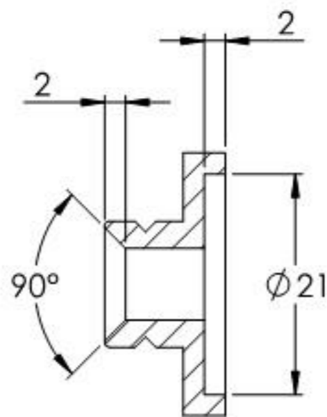
SCHNITT C-C
